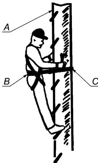
А - крепление; В - привязь; С - строп для системы позиционирования (применяется для работ на столбах)
