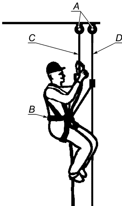
A - крепление; B - привязь; C - рабочий канат; D - страховочный канат
